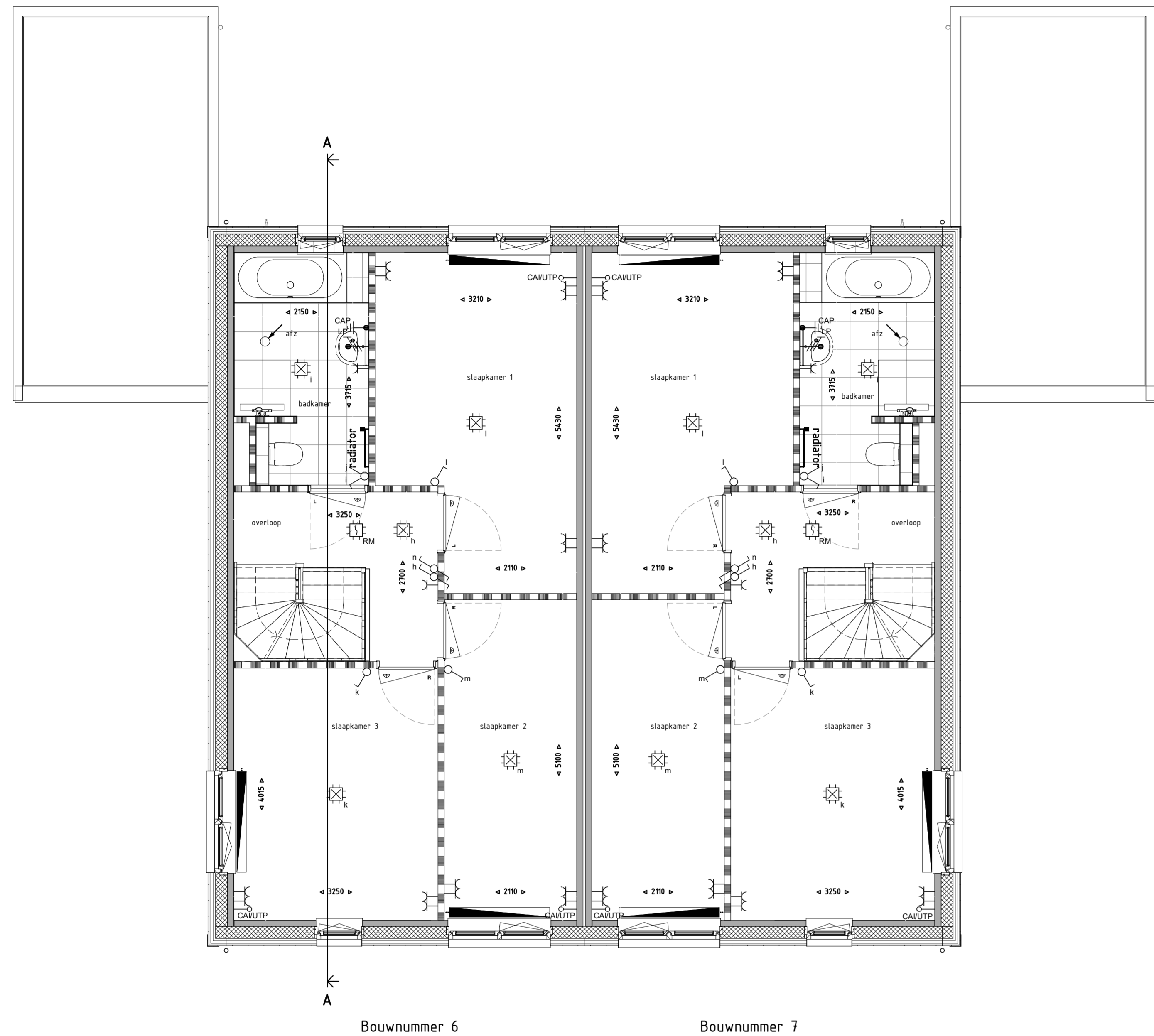
1E VERDIEPING 1 : 50
