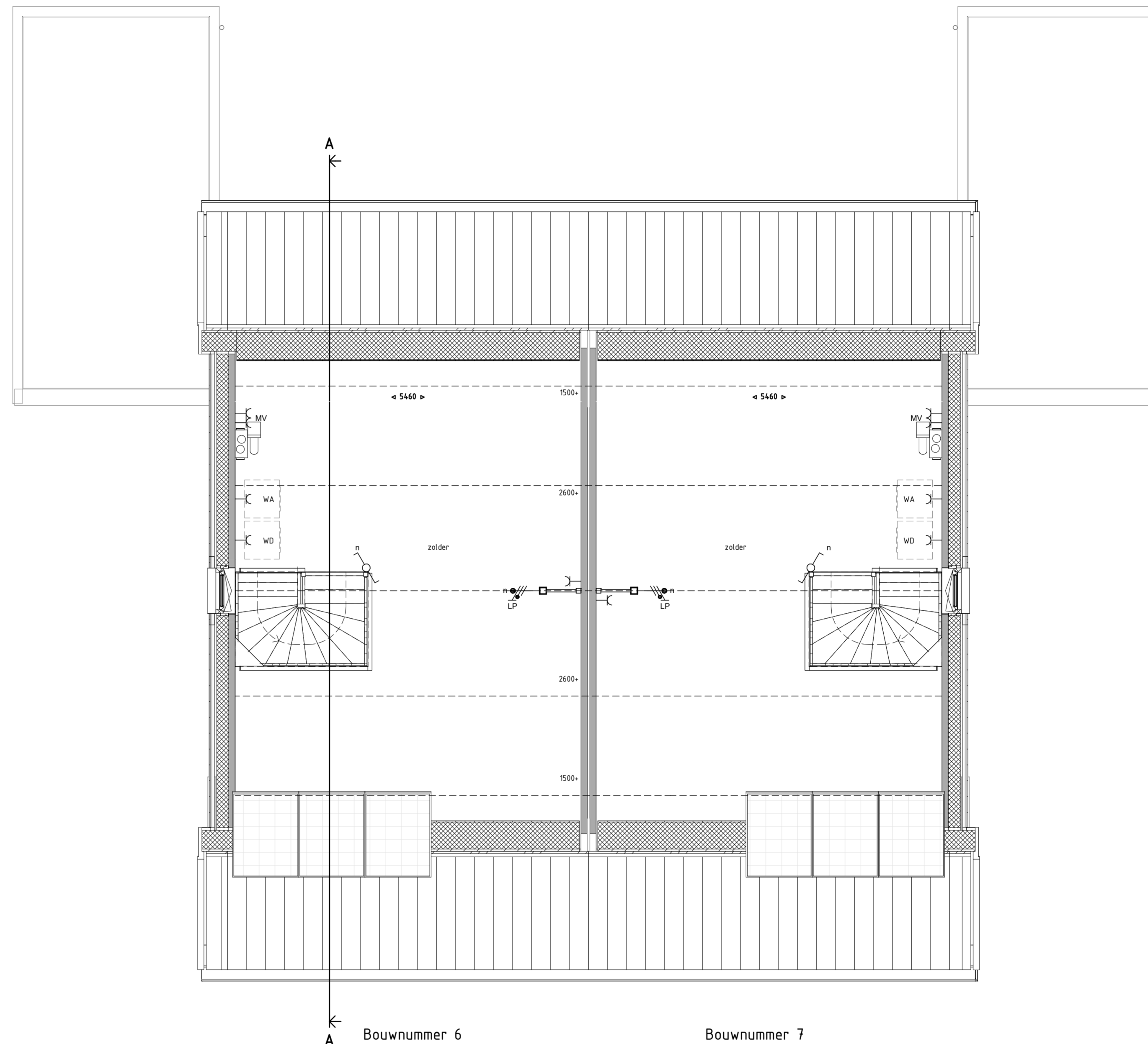
2E VERDIEPING 1 : 50
